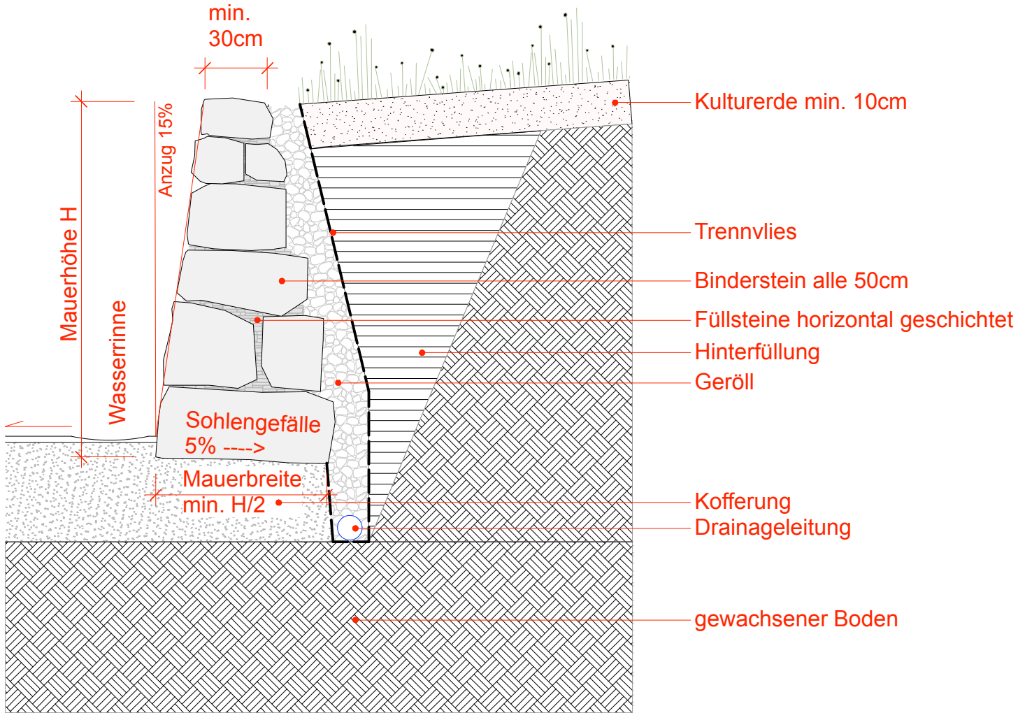
Querschnitt
